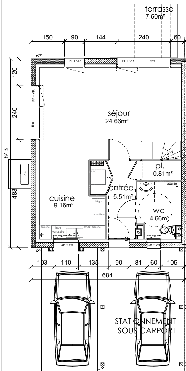
Rez-de-Chaussée
