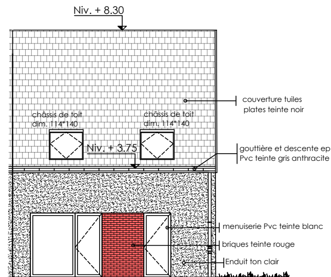
Façade Arrière
