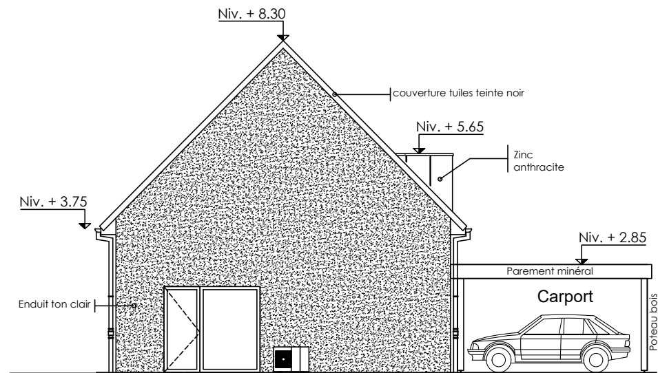
Pignon Gauche
